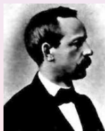
Christoffel
