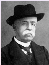
Ricci
