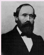
Riemann
